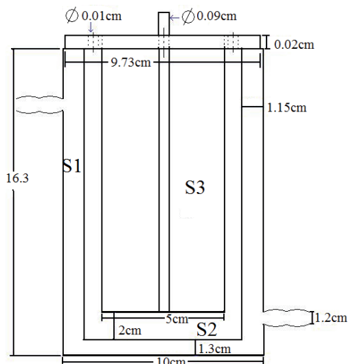
Fig. 2. Reactor Fotocatalítico.
