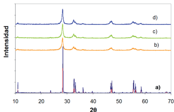
Fig.6. Difractograma del polimorfo de baja temperatura (L-Bi 2 MoO 6 ), JCPDS No. 01-084-0787 -Keochilinite- Bi 2 MoO 6 (color rojo). a) estado sólido, y activado mecánicamente b) 5 horas, c) 11 horas y d) 21.5 horas.
