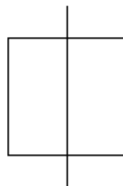
Fig. 1. El rectángulo es simétrico respecto a la línea que lo divide en dos partes iguales.
