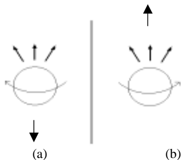
Fig. 3. En (a) la flecha inferior indica la dirección del espín y las flechas superiores la dirección en la que salen los electrones producto del decaimiento. En (b), que es la imagen especular de (a), la flecha superior indica la dirección del espín y las otras flechas la dirección de los electrones. El proceso (b) no se observa en la naturaleza.
