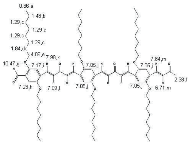
Fig. 5. Estructura del producto de condensación aldólica y asignación de picos de 1 HNMR aldehído.
