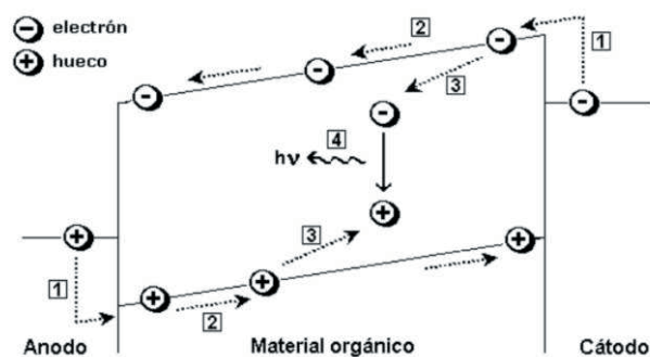
Fig. 2. Etapas básicas del fenómeno de electroluminiscencia en materiales orgánicos. 1. Inyección de portadores de carga, 2. Transporte de portadores de carga, 3. Formación
