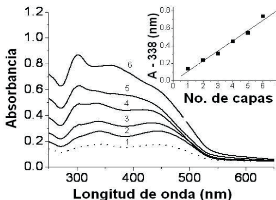
Fig. 7. Espectros UV-Vis de muestras con PBTA con diferente número de capas (hasta 6, se indican en figura), inserto; gráfica de la absorbancia a 338 nm normalizada con respecto al valor a 650 nm, vs. número de capas (cada capa es doble, una a cada lado del sustrato).
