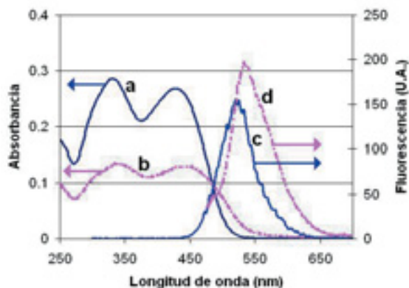
Fig. 6. Espectros de absorción U.V. Vis. del PBTA a) en disolución, b) en película y sus espectros de fluorescencia, c) en disolución y d) en película.
