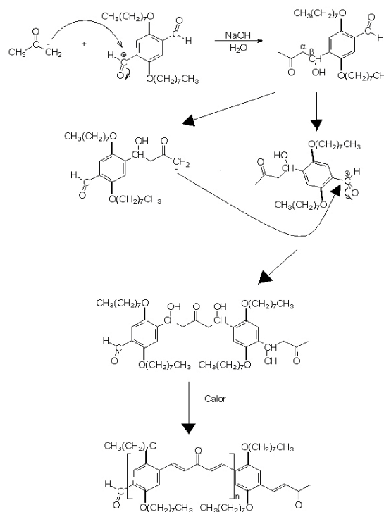
Fig. 3. Ruta de síntesis mediante condensación aldólica de sustancias con moléculas conjugadas.
