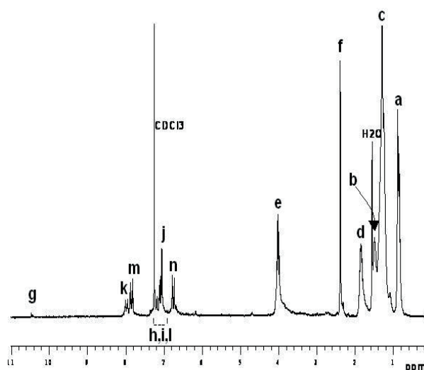
Fig. 4. Espectro 1 HNMR del producto de condensación aldólica, las letras sobre los picos corresponden a su asignación la cual se muestra en la figura 5.
