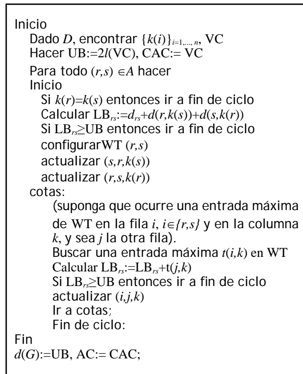
Fig. 4. Algoritmo de Dvir-Handler.
