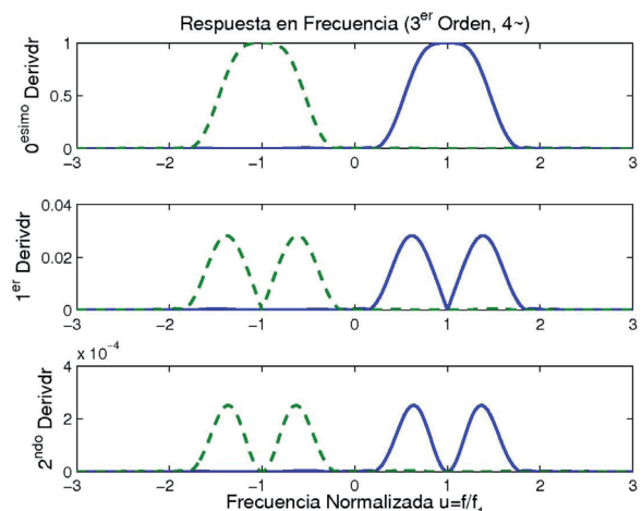
Fig. 4. Respuesta en frecuencia del estimador Taylor-Fourier de 4 ciclos, usando WLS con ventana de Kaiser ( \kappa = 3 , \alpha = 8 ) (línea continua), y sus complejos conjugados (línea discontinua).
