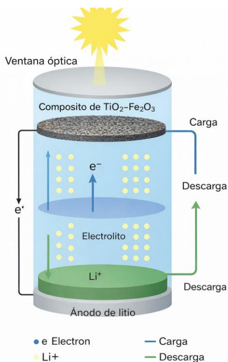
Fig. 2. Configuración de fotobaterías de ion-litio.
