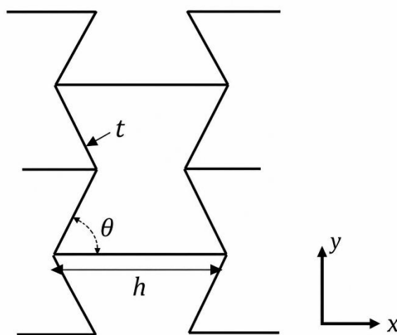
Fig. 3. Celda unitaria auxética reentrante y parámetros geométricos principales.
