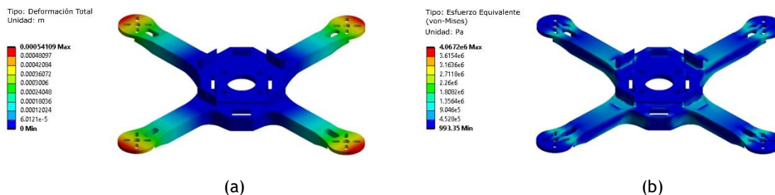
Fig. 3. Análisis estructural del cuadrirrotor: (a) Deformación total. (b) Esfuerzo equivalente.
