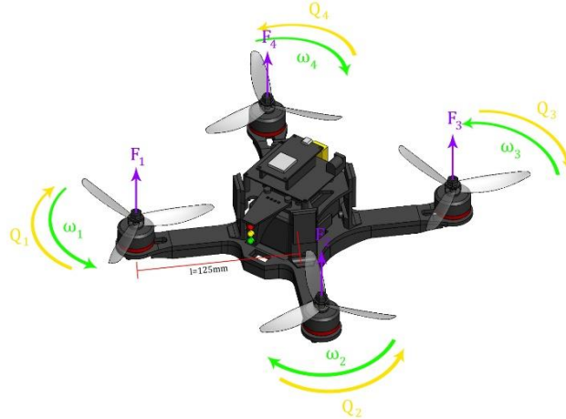
Fig. 5. Convención de fuerzas y momentos del cuadrirrotor.
