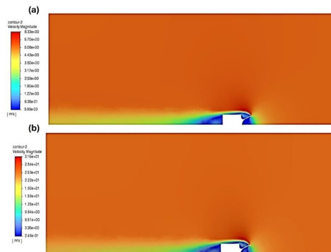
Fig. 4. Resultados numéricos de velocidad en micro turborreactor SR-30.
